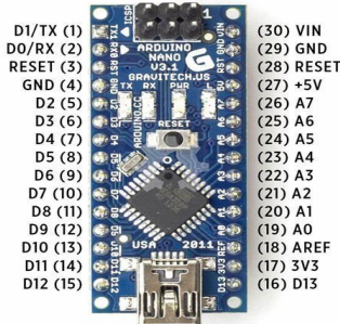
Fig 1. Arduino nano
