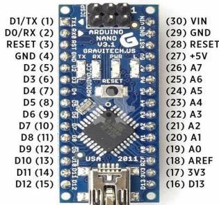
Fig 1. Arduino nano
