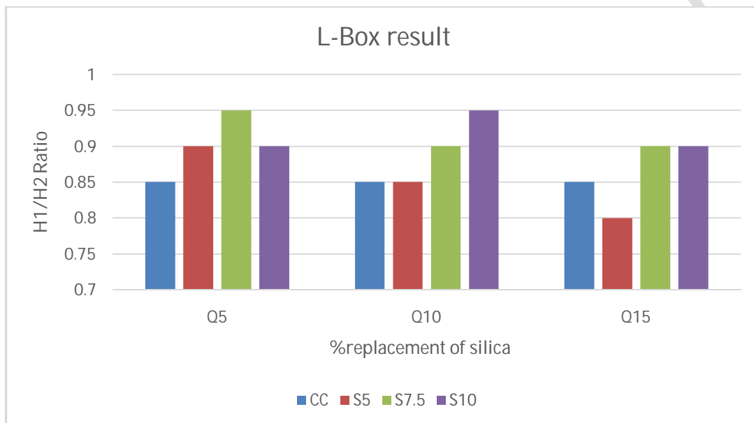
Fig. 7. L-Box test result [19]
