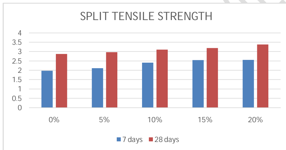
Fig.16. Split tensile strength test results [28]
