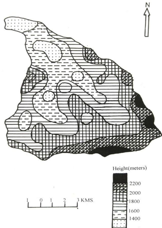
Fig.4. Absolute Relief Map
