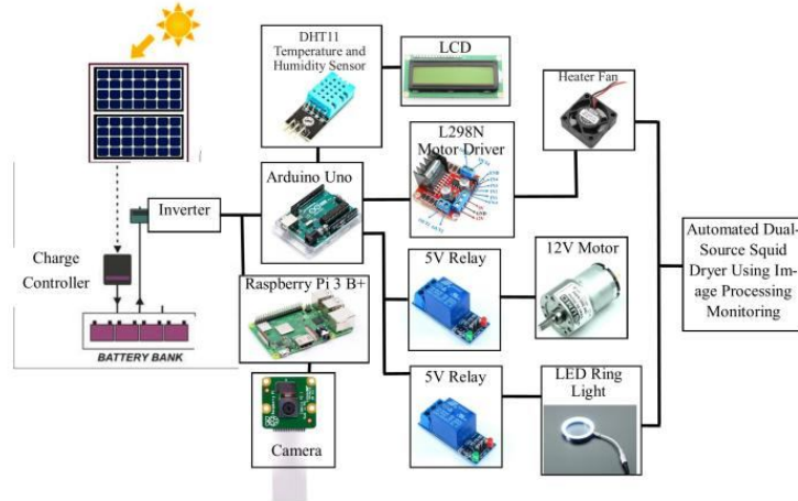
Fig. 11. Schematic
