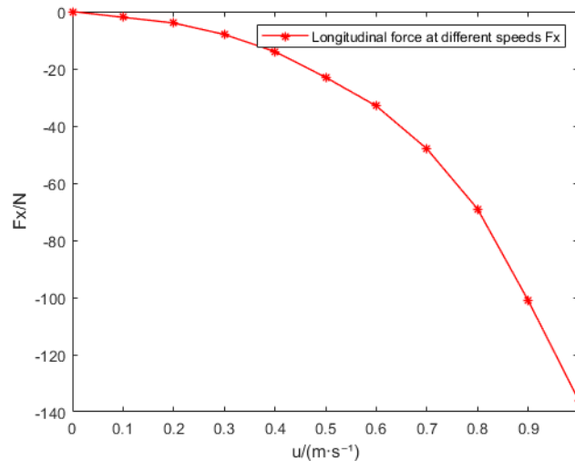
Fig 13 F_x in longitudinal motion
