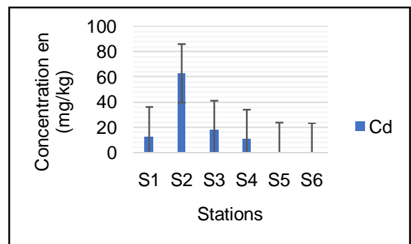
Fig. 2-d : Cadmium distribution
