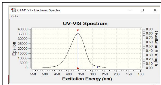
Chloroform 6-31+G(d)
