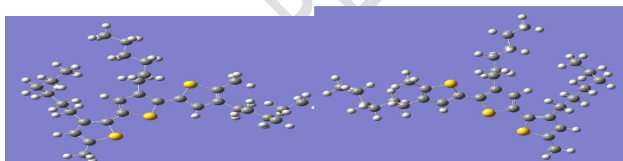
Anionic P3HT
