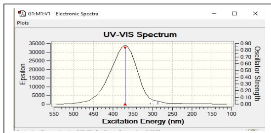
Chloroform 6-31++G(d,p)
