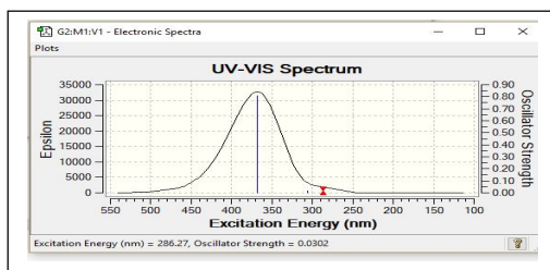
Methanol 6-31++G(d,p)
