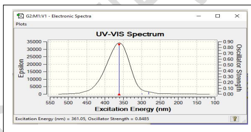
Chloroform 6-31+G(d)
