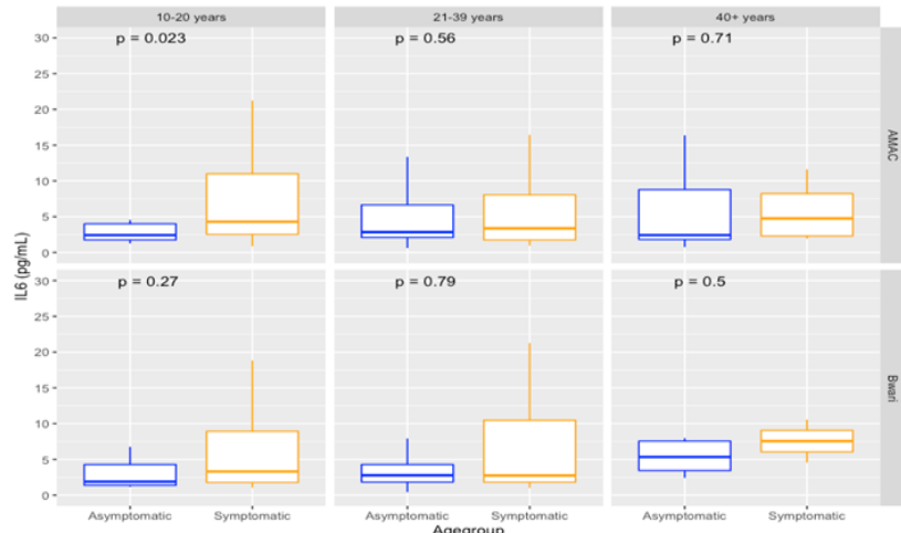
IL-6 (pg/mL)
