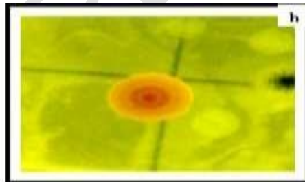
Solubilisation de BN avec du FePO 4
