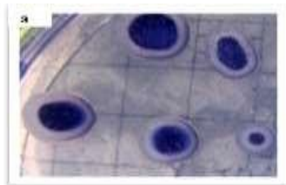
Solubilisation BN avec du CaPO 4
