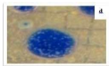
BG12 pas de halo de solubilisation
