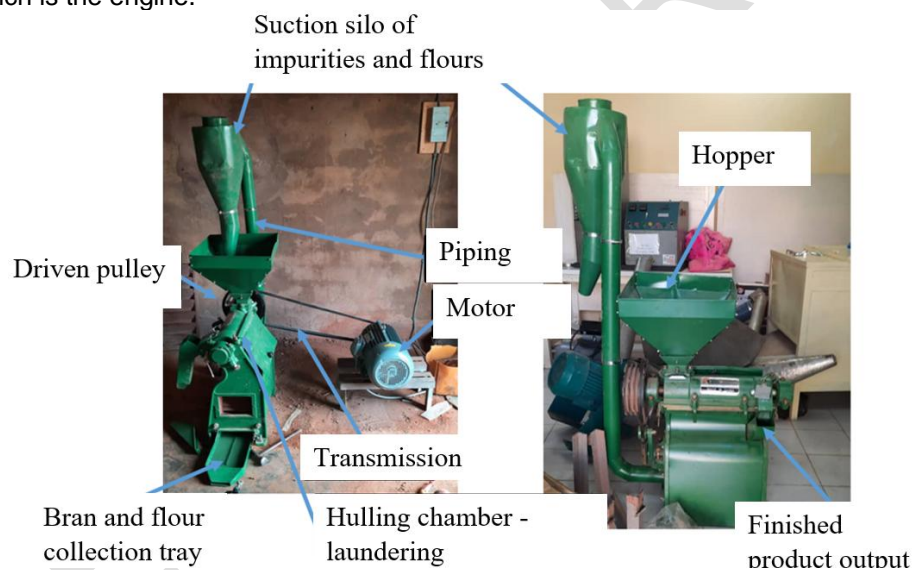
Fig. 7. Cereal husker
