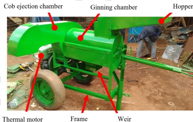
Fig. 1.ZEKEDA maize sheller
