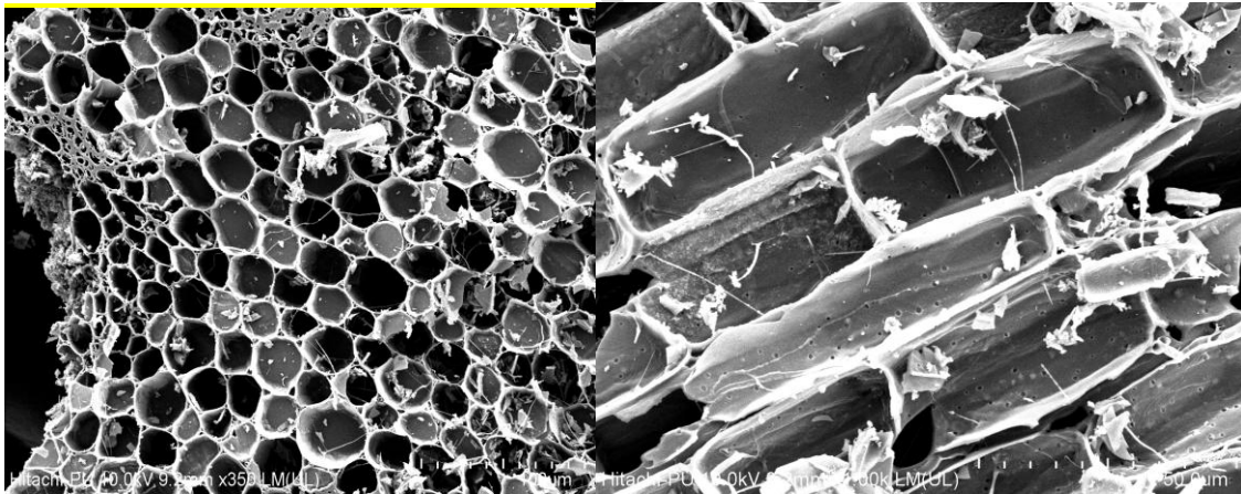
Fig.1 FE-SEM images of biochar
