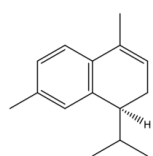
(d) \alpha -calcorene
