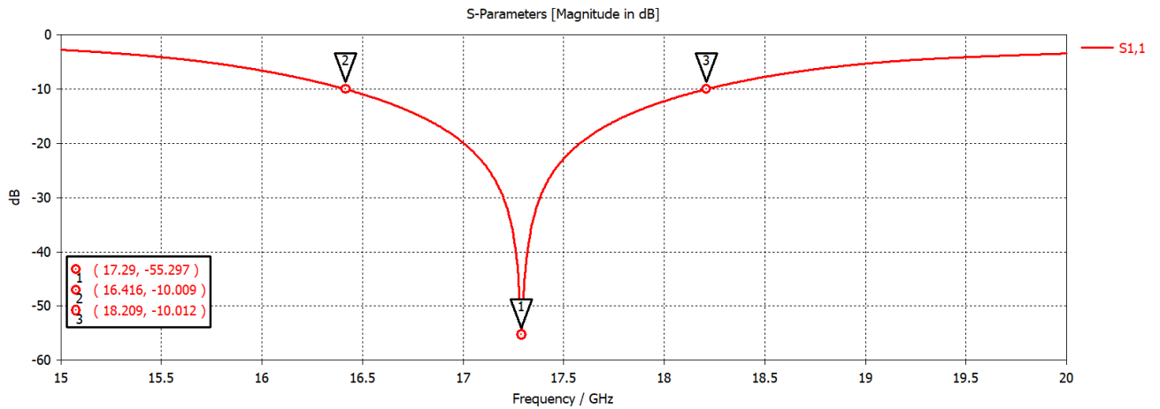
Fig. 3. Return Loss (S11-parameters)
