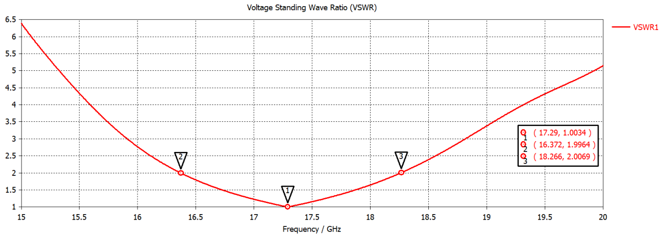
Fig. 4. VSWR
