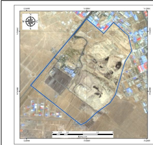
2019-09-17 Landsat8 image
