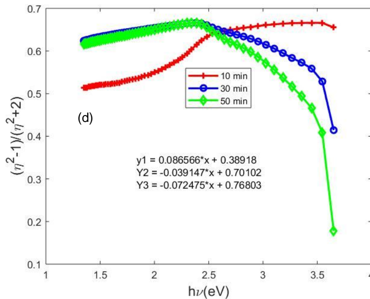
Fig8 (d) \frac{\eta^2-1}{\eta^2+2} Versus h\nu (eV) Fig8 (a)
