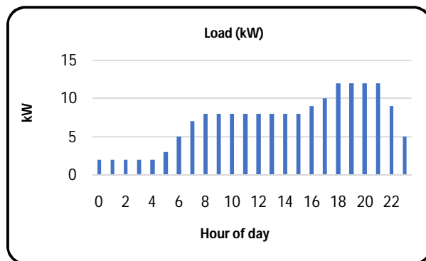
Fig. 21. Load profile
