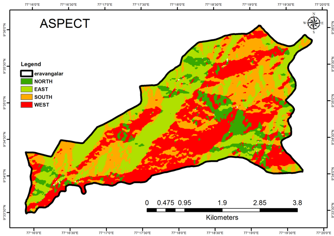
Fig. 3. Aspect Map
