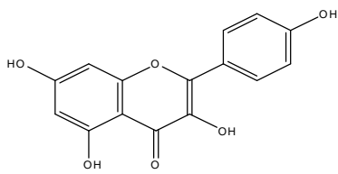
Kaempferol
