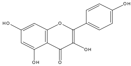
Kaempferol
