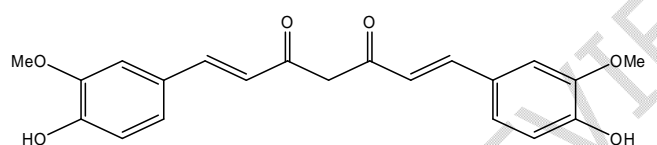
Curcumin
