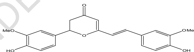
cyclocurcumin
