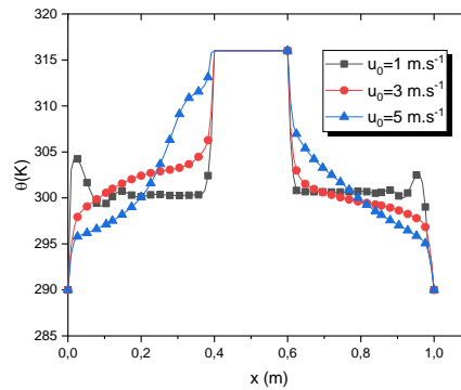
Figure 18: Profils de la température en fonction de x pour différentes valeurs du module de la vitesse des parois verticales en sens opposés
