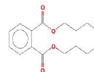
Dibutyl phthalate
