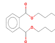
Dibutyl phthalate
