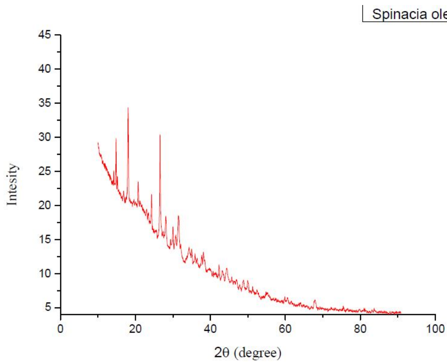
Fig. 1(d) XRD pattern for Spinacia oleracea
