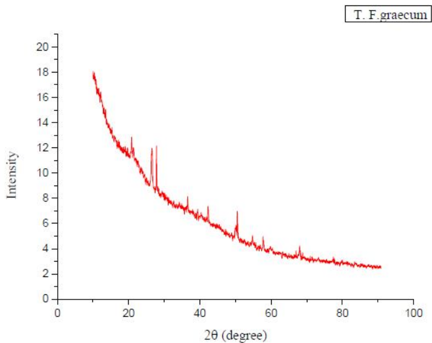
Fig. 1(c) XRD pattern of T. F. Graecum
